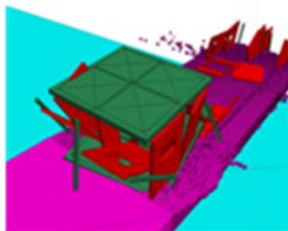
図4 土砂災害シミュレーション 3)
