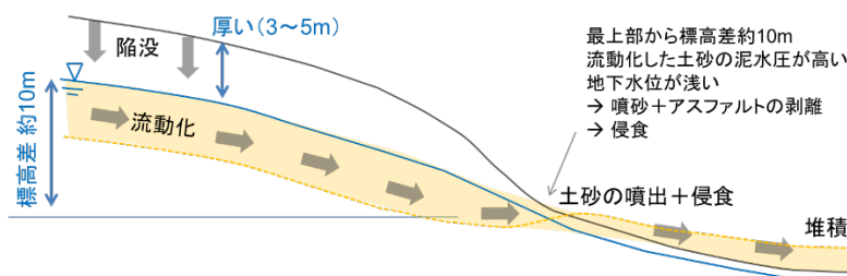
図1. 札幌市清田区里塚一条の液状化による被災メカニズム
