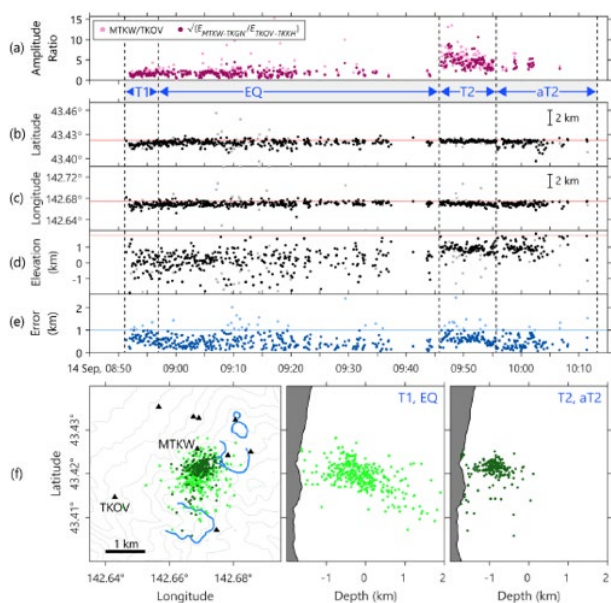
図 1. 2020 年 9 月の地盤変動イベントで見られた地震活動域の浅部への移動 (Permana and Aoyama, 2022).
