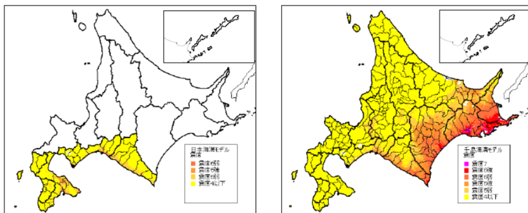
日本海溝(三陸・日高沖)モデル
