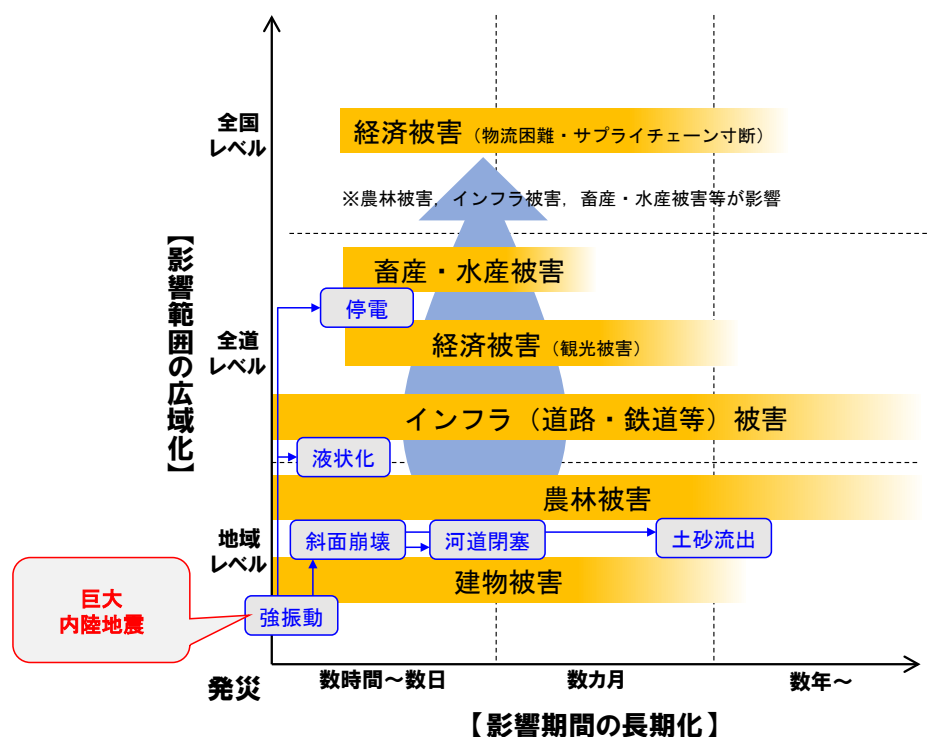
図 2.4 北海道胆振東部地震における現象の連鎖発生と被害の広域複合化のイメージ
