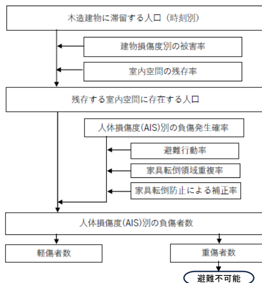
図 3.7 人的被害計算フロー
