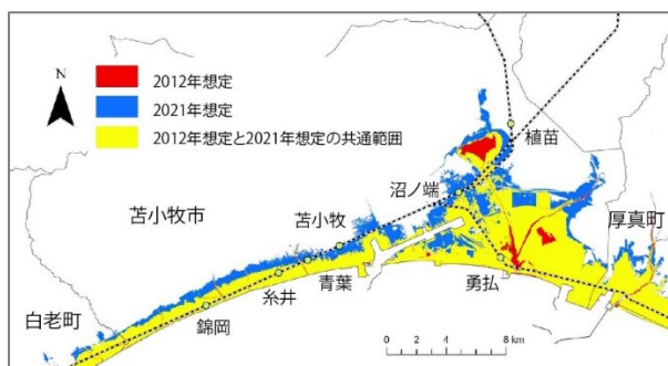
図1 2012年と2021年の津波浸水想定
