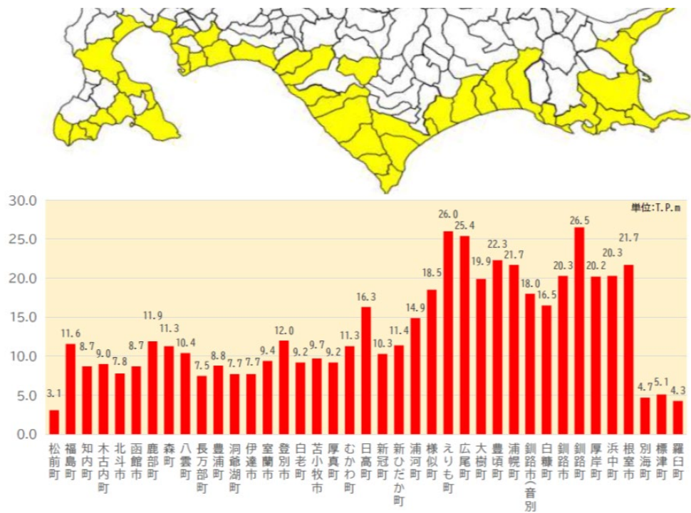
図 3.5 北海道公表の最大津波高
