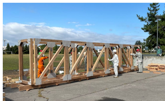
写真-7 木製緊急架設橋の架設実験
