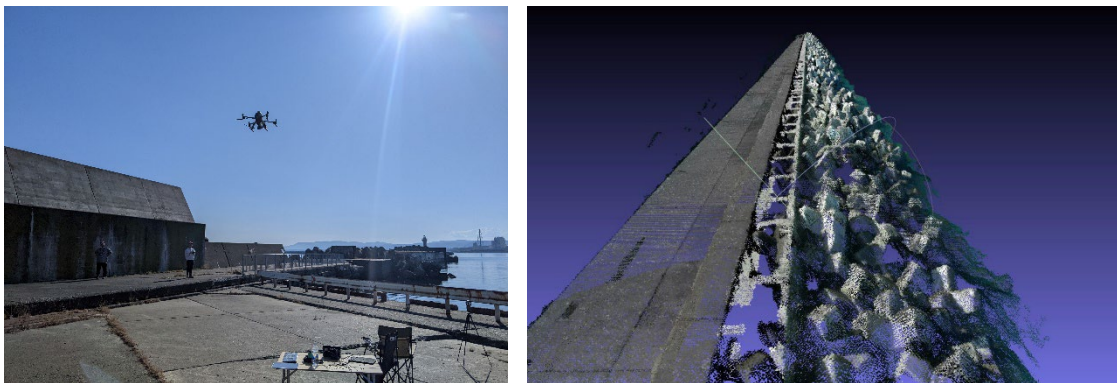
図 1. (左) 実証実験の様子。(右) 提案手法によって得られた防波堤の 3 次元点群。ここからアルゴリズムに従って消波ブロックの欠損量を定量的に評価することができる。
