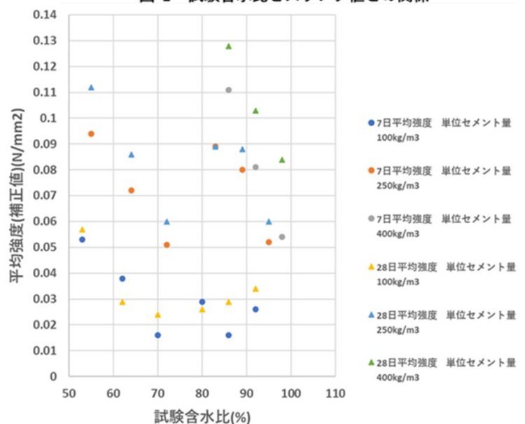
図-2 試験含水比と平均強度との関係
