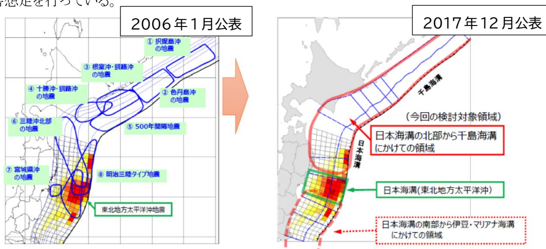
図 3.1 当該海域における地震断層モデル
