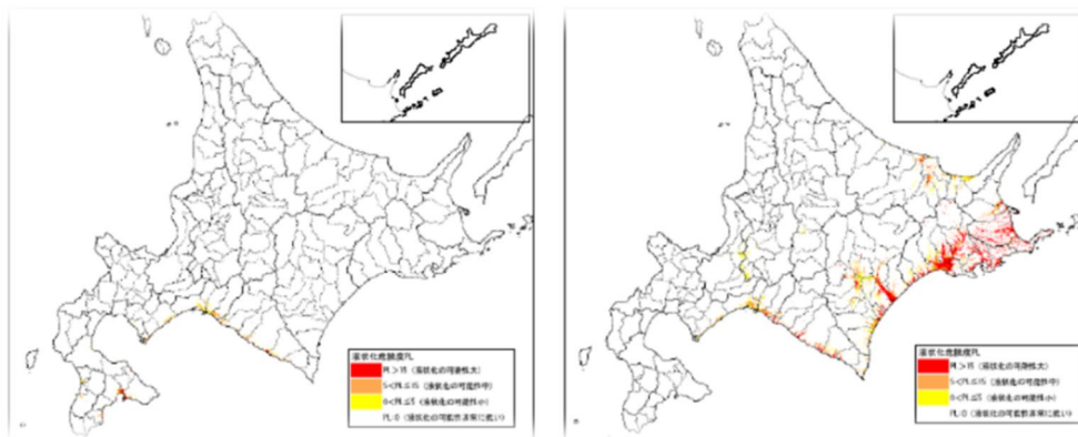
日本海溝モデルによる土砂災害危険ランク
