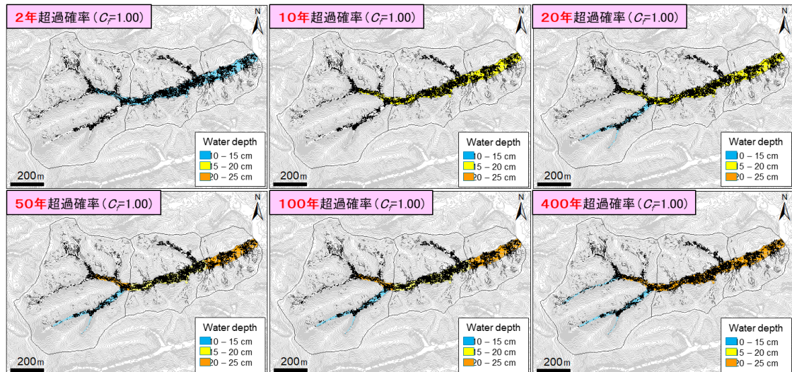
図 1. 降雨の超過確率規模に応じた水深変化。水深が深くなるほど河道内に堆積している流木の移動割合が大きくなり二次移動による流木ハザードが高くなる。Koi et al. (2022) を加筆修正
