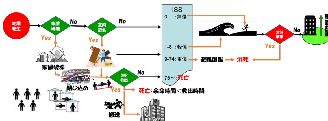
図 3.8 地震と津波同時発生による人的被害算定シナリオ
