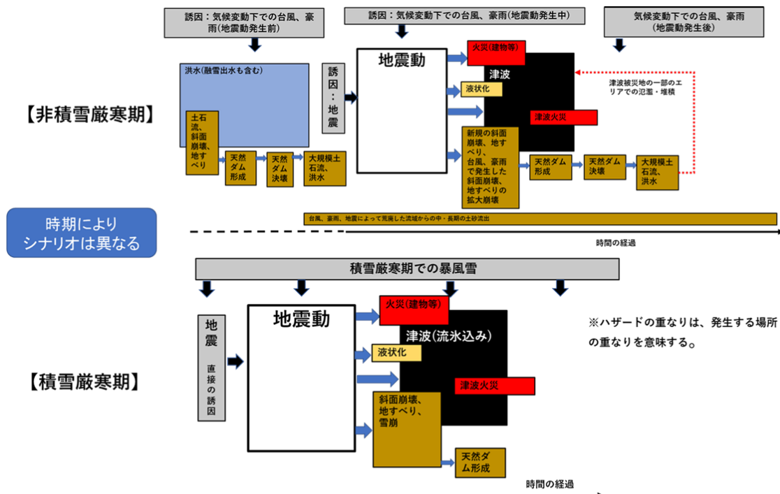
図1.4 広域複合災害をもたらすハザードと災害の連鎖・複合化プロセスの想定事例
