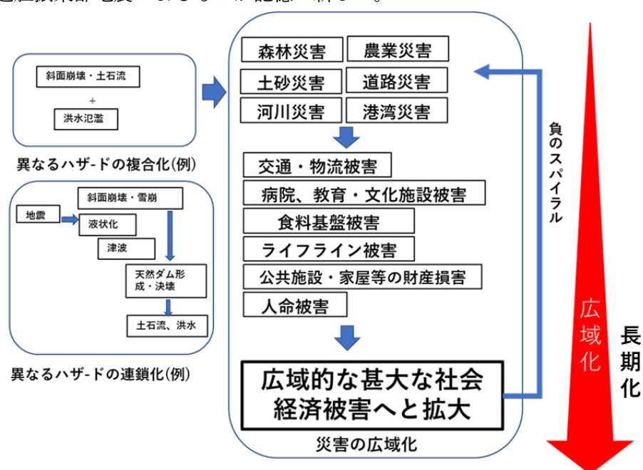
図1.1 広域複合災害をもたらすハザードと災害の複合化、連鎖化、広域化、長期化
