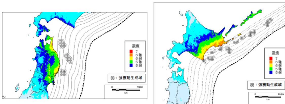
日本海溝(三陸・日高沖)モデル
