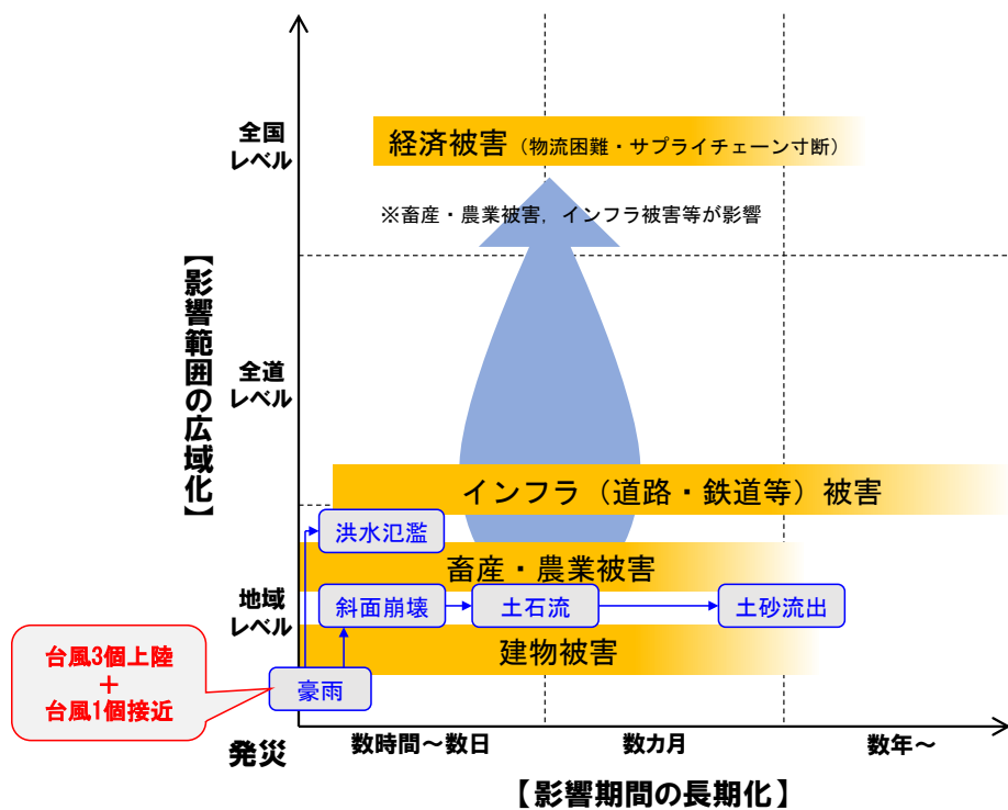
図 2.2 2016 年北海道東部豪雨災害における現象の連鎖発生と被害の広域複合化のイメージ
