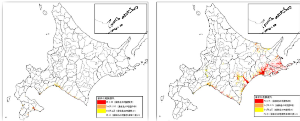
日本海溝モデルによる液状化危険度
