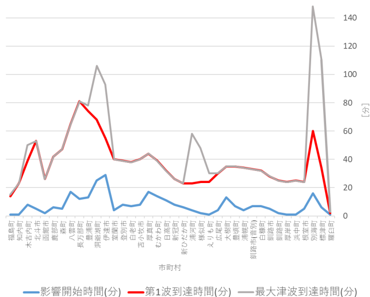
図 3.6 北海道公表の津波到達時間
