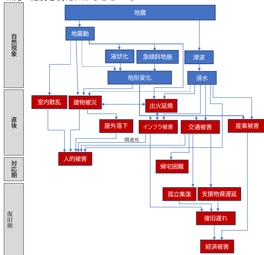
図 3.9 被害算定式にみる各事象の複合化プロセス
